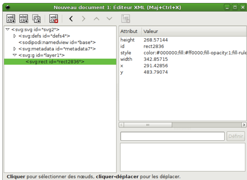
FIGURE 3-1 L'éditeur XML
