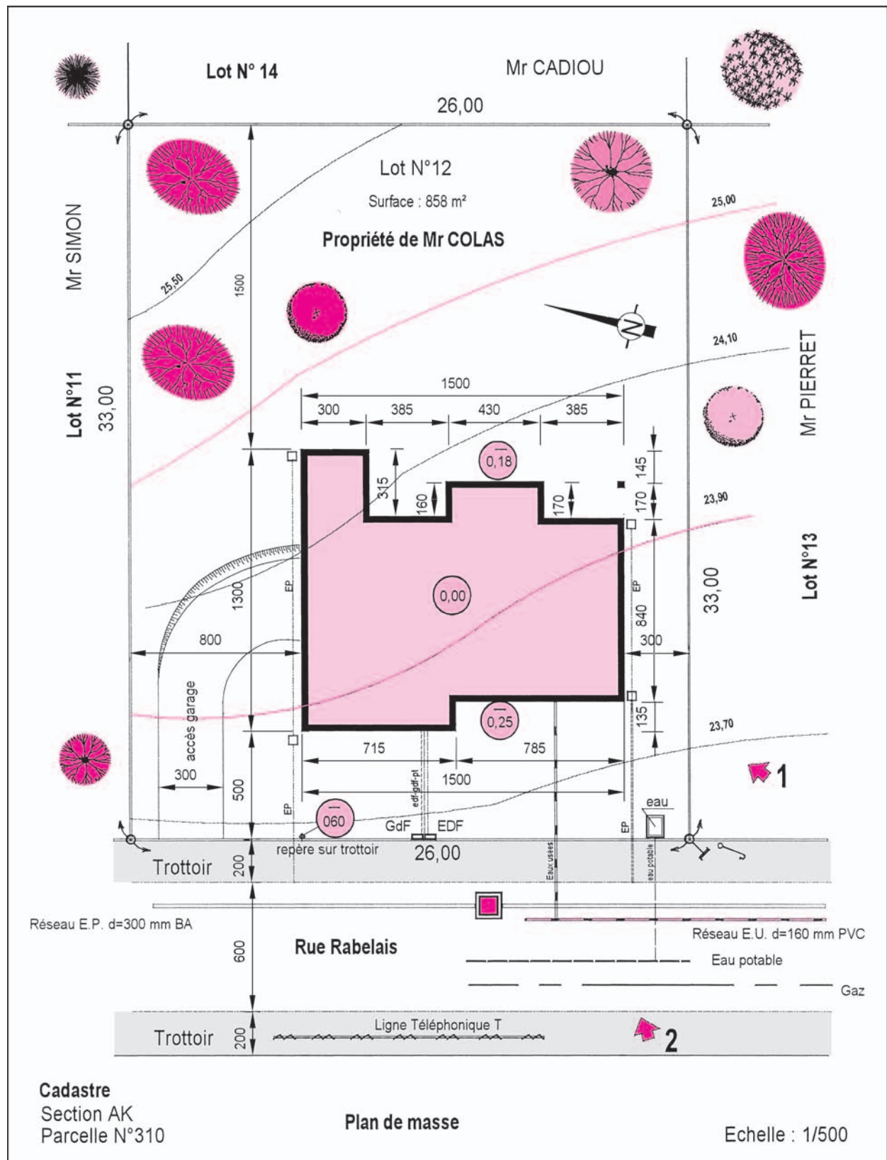
Fig. 17 : Plan de masse avec les cotes d'implantation des murs extérieurs
