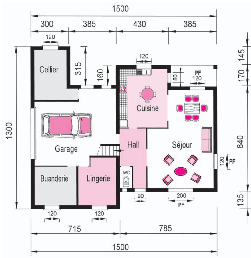
Fig. 18 : Schéma de principe d'avant-projet du rez-de-chaussée
