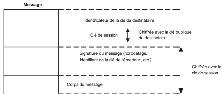
Figure 8.10 Format d'un message PGP
