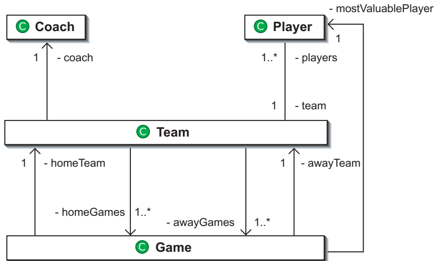
Figure 2-4 Diagramme de classes exemple
