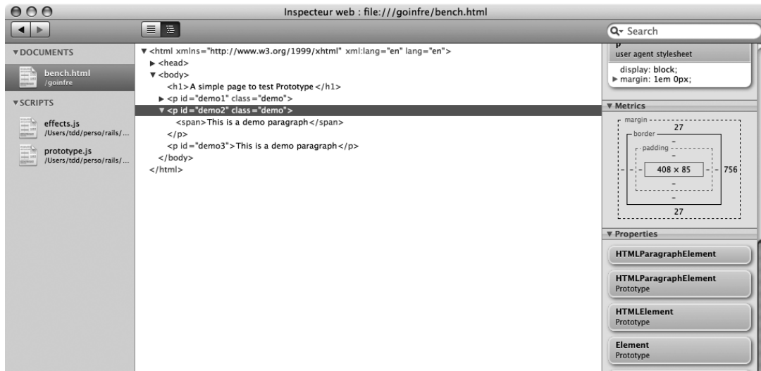
Figure D-10 L'inspecteur web de Safari 3 affiche les métriques d'un élément
