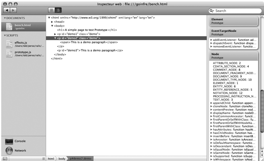
Figure D-11 L'inspecteur web de Safari 3 affiche le DOM d'un élément
