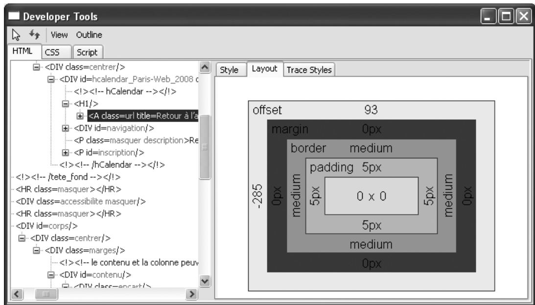
Figure D-19 L'outil de développement intégré à IE8 et son onglet Layout
