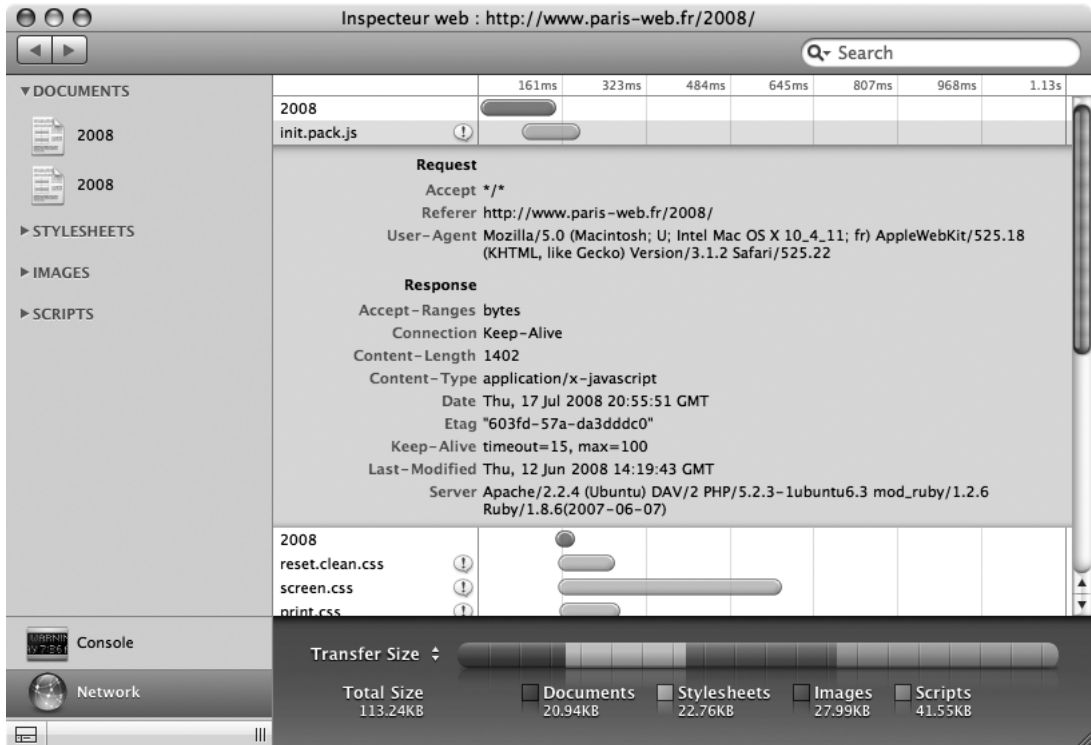
Figure D-14 Inspecteur de vitesse réseau sur Safari 3 avec examen des en-têtes
