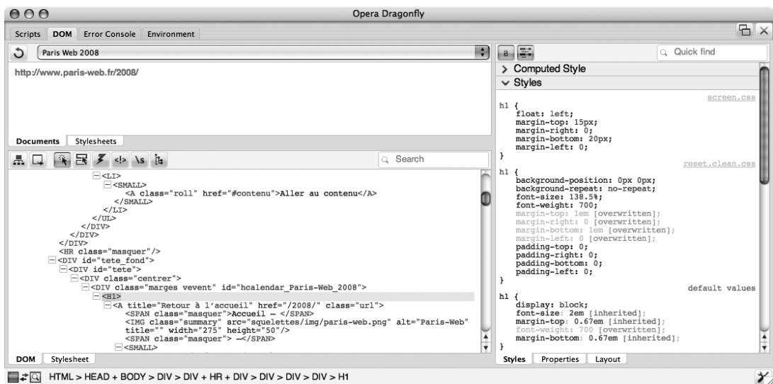
Figure D-22 La vue DOM d'Opera Dragonfly : un parfum de Firebug...
