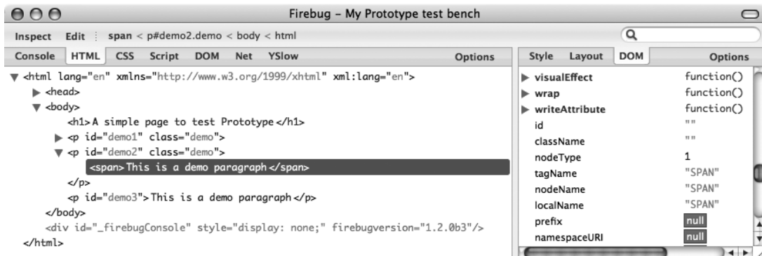
Figure D-3 L'inspecteur DOM pour l'élément sélectionné dans Firebug
