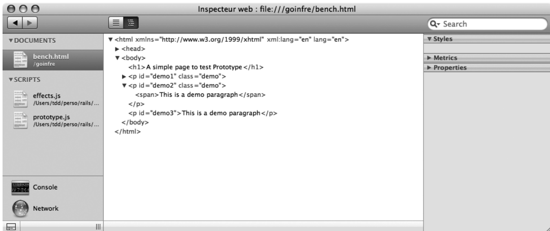
Figure D-8 L'inspecteur web en mode arborescent.
