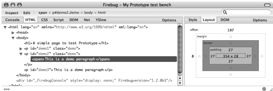
Figure D-2 L'onglet Layout de Firebug se révèle vite incontournable !
