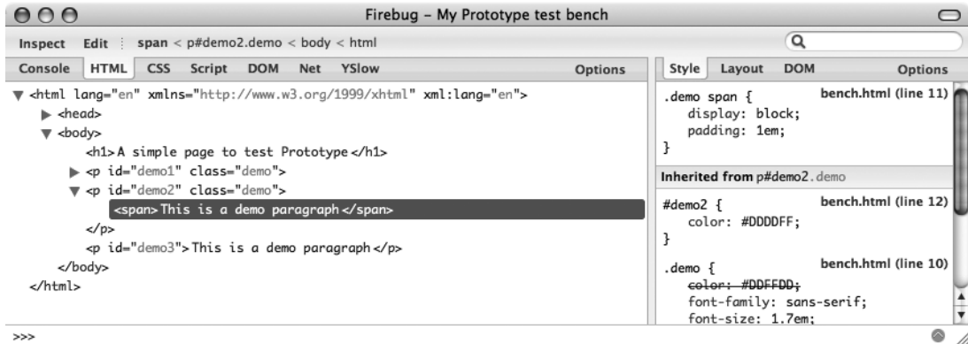
Figure D-1 L'inspecteur de code source de Firebug, en mode « style »
