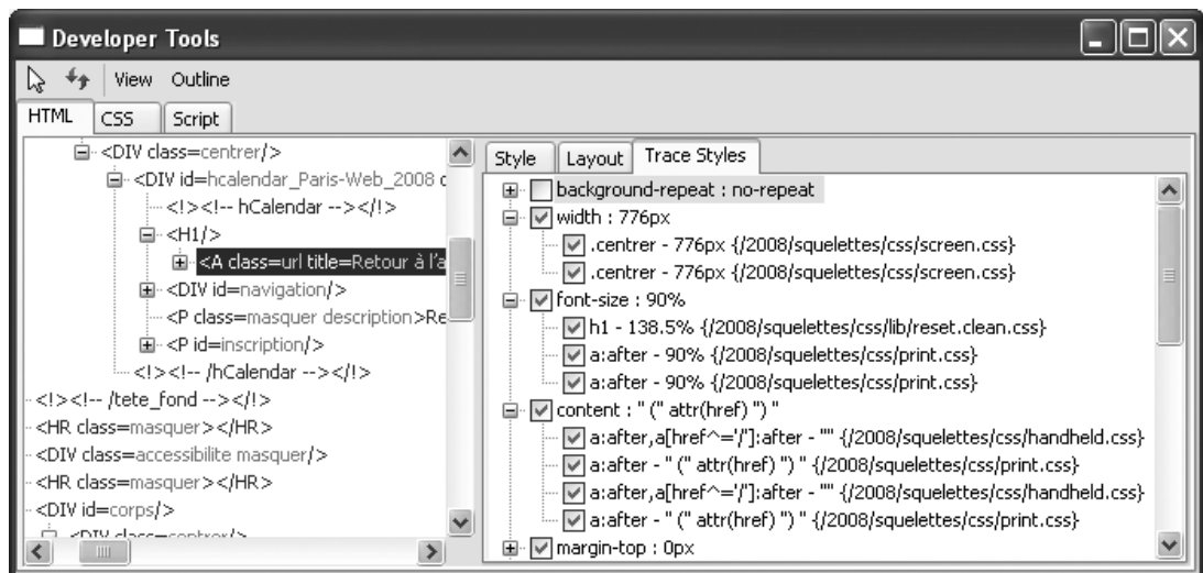
Figure D-20 L'outil de développement intégré à IE8 et son onglet Trace Styles
